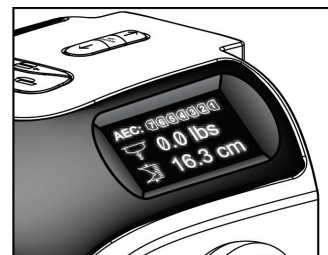
Figur 10: Komprimeringsanordningens display
