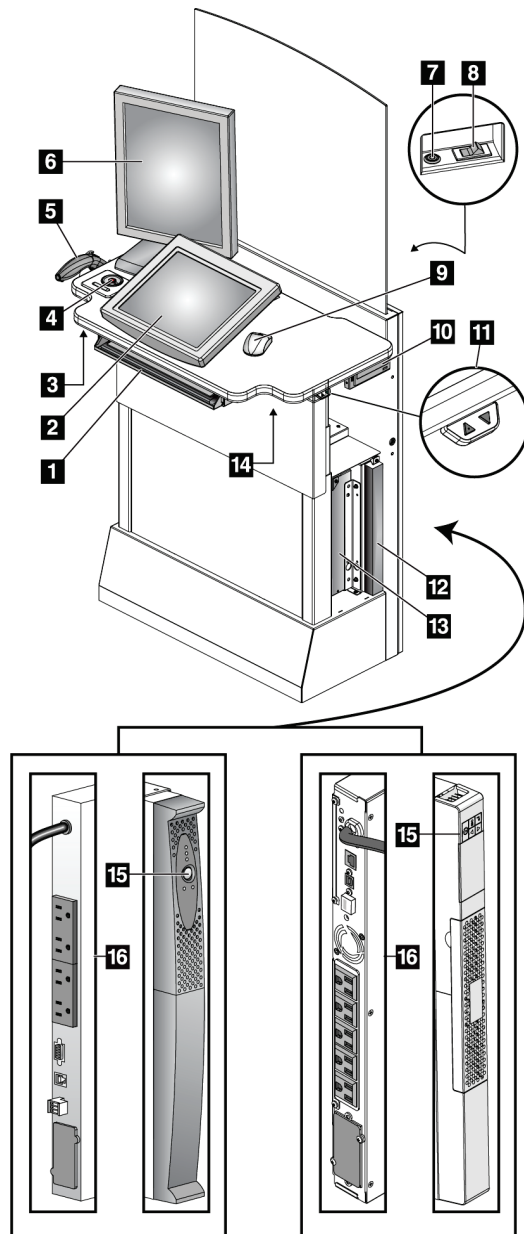
Figur 6: Kontroller och displayer på standardbildtagningsstationen
