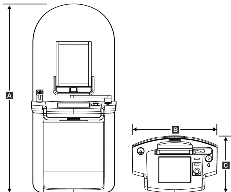
Figur 68: Mått på Premium bildtagningsstation
