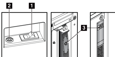
Figur 15: Strömknappar på standardbildtagningsstation
