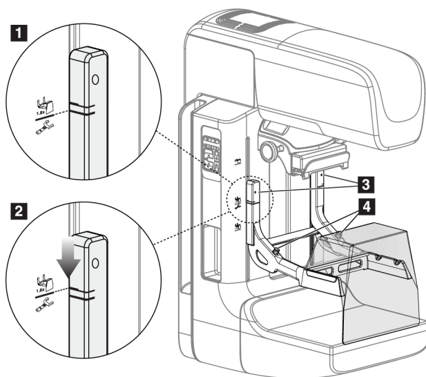
Figur 53: Installera förstoringsstativet
