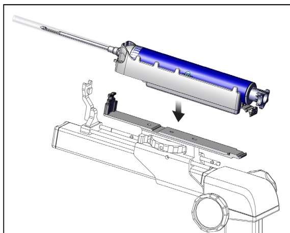
Εικόνα 63: Προσάρτηση της συσκευής βιοψίας
