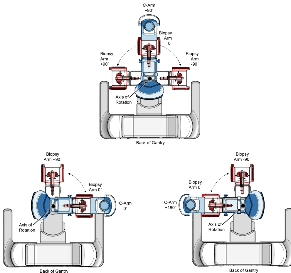
Εικόνα 44: Γωνίες περιστροφής βραχίονα βιοψίας
