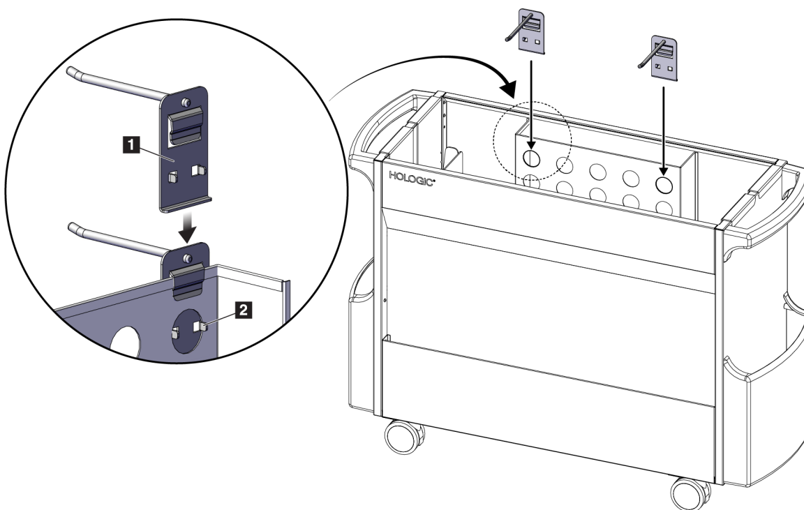
Εικόνα 64: Τοποθέτηση άγκιστρων επιθεμάτων
