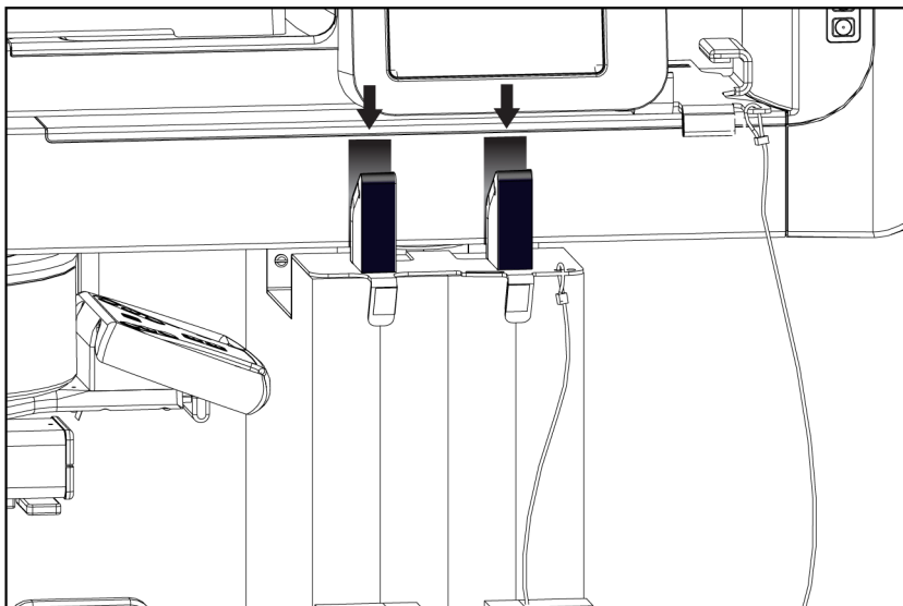
Εικόνα 89: Ευθυγράμμιση σημάνσεων του C-arm με τη βάση του C-arm
