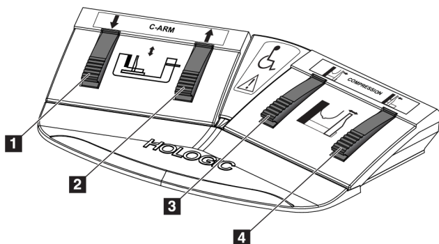
Obrázok 9: Pedál – podrobný prehľad
