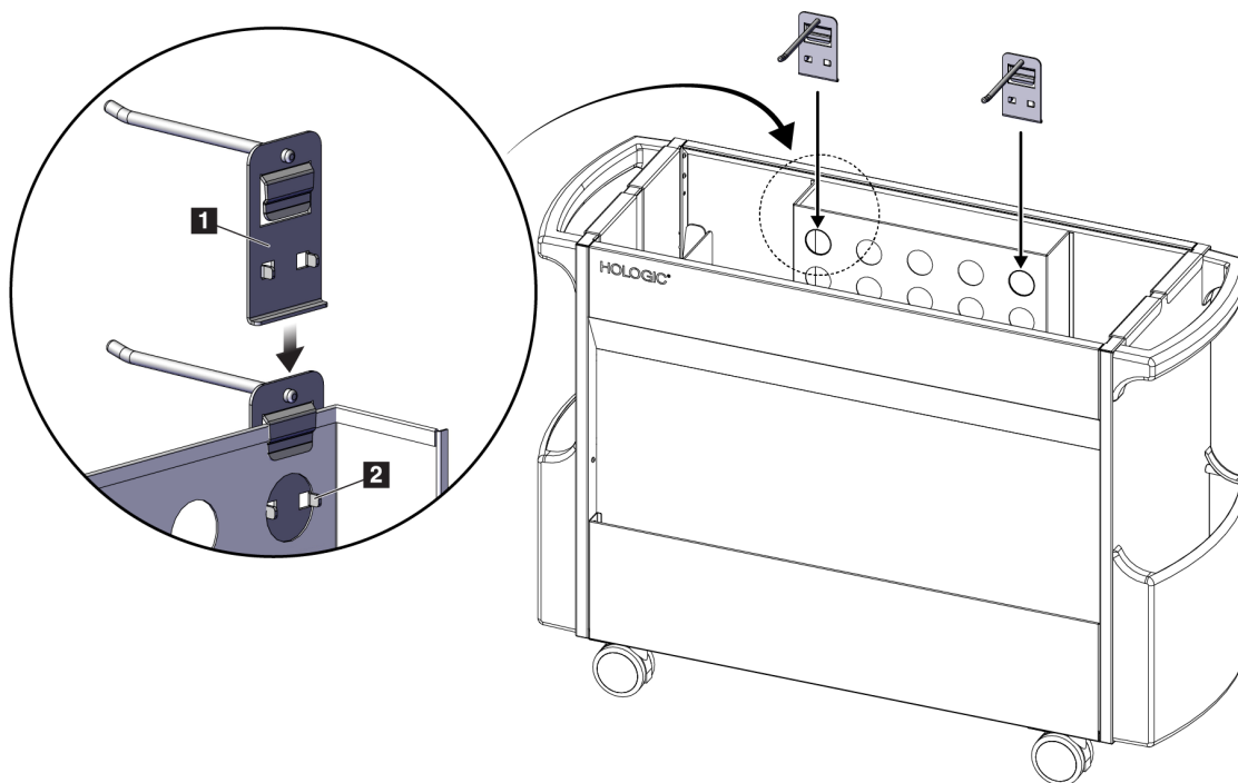
Obrázok 64: Inštalácia vešiaka na podložky
