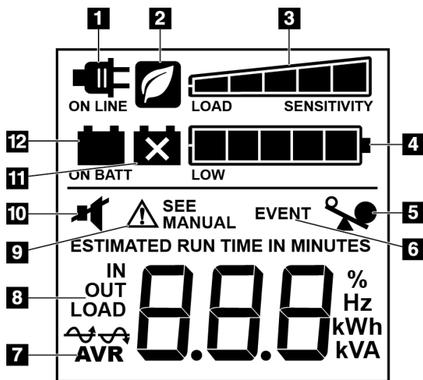
Obrázok 84: Displej LCD zdroja UPS
