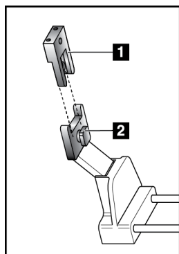
Obrázok 61: Ako inštalovať ihlové vodiče
