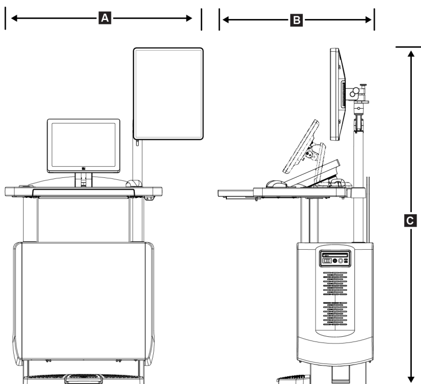
Figuur 106: Afmetingen mobiel universeel verwervingswerkstation
