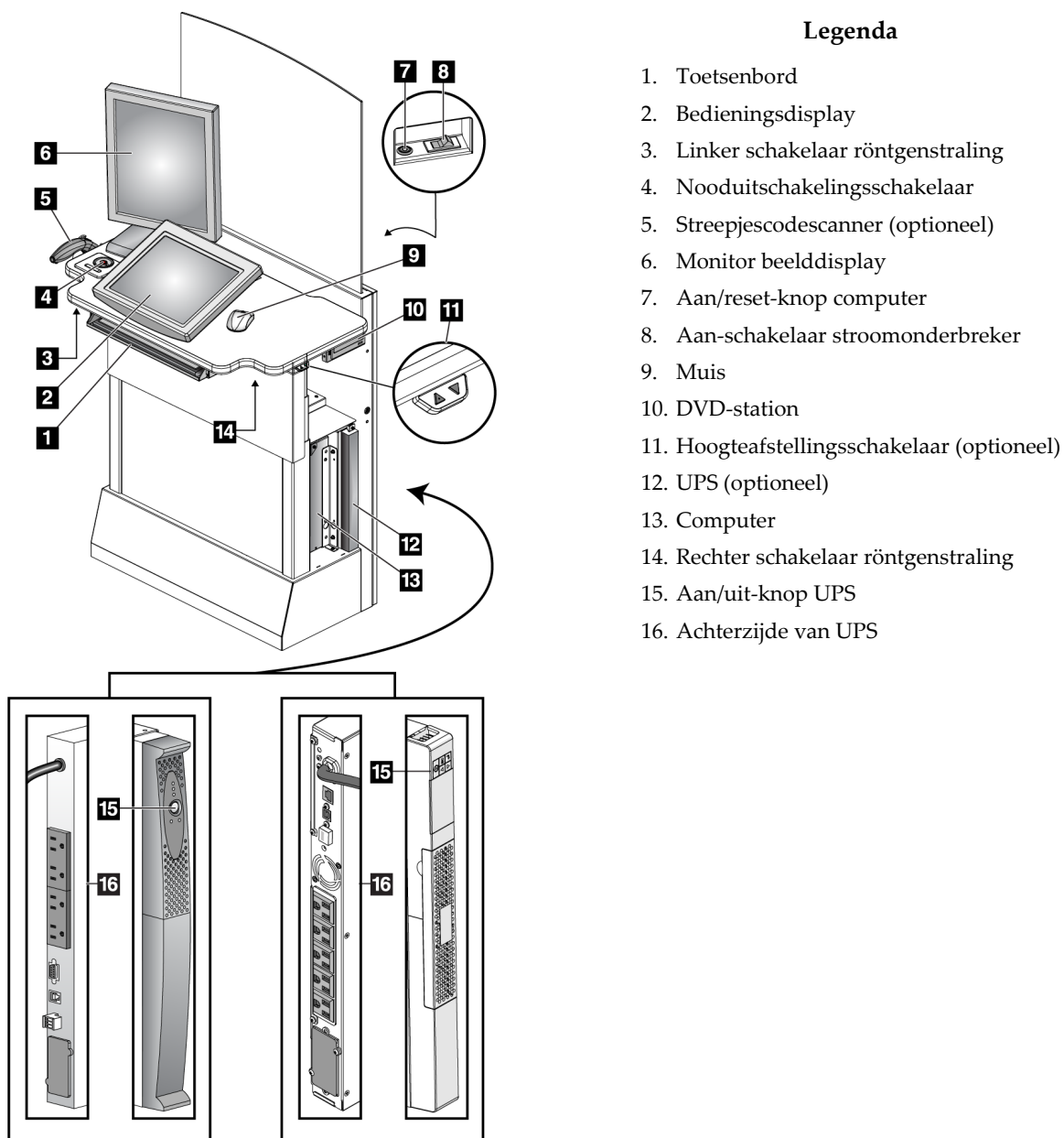
Figuur 15: Bedieningselementen en displays van het Standaard verwervingswerkstation
