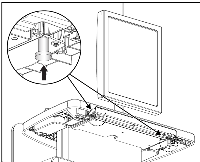
Figuur 109: Vergrendelingsknop toetsenbordlade, rechts of links (Universeel verweringswerkstation)
