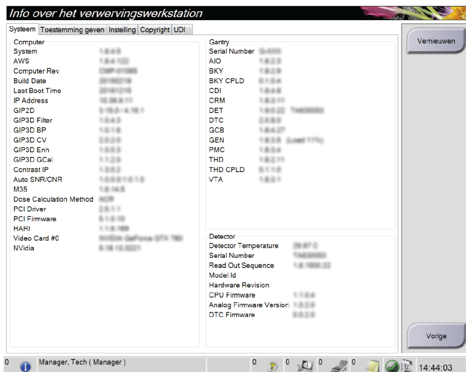
Figuur 79: Tabblad Systeem van het scherm Info (het verwervingswerkstation)
