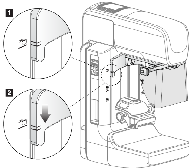
Figuur 64: Het intrekbare gezichtsscherf uitlijnen met de C-arm
