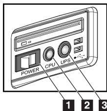
Figuur 17: Aan/uit-knoppen Universeel verwerfingswerkstation
