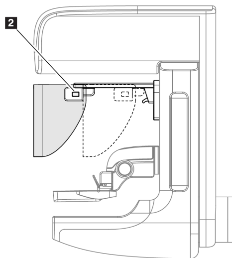
Figuur 66: Bediening van het gezichtsschermb
