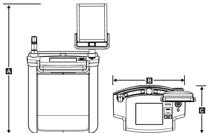
Figuur 107: Afmetingen Premium mobiel ververingswerkstation
