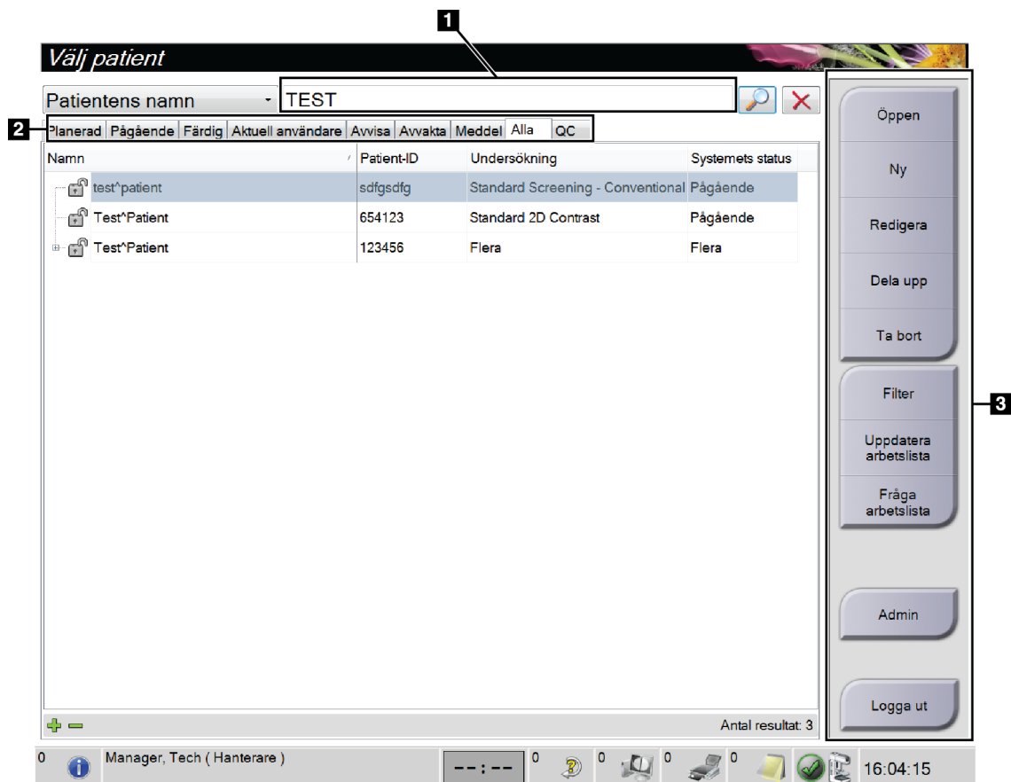
Figur 30: Välj patientskärm
