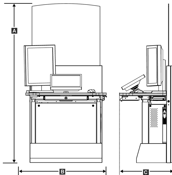
Figur 105: Mått på standard bildtagningsstation
