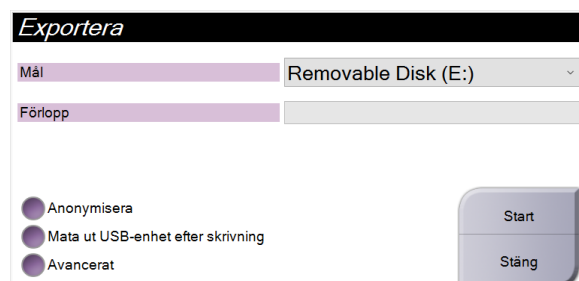
Figur 45: Dialogrutan Exportera
