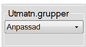
Figur 42: Fältet Utmattn.grupper
