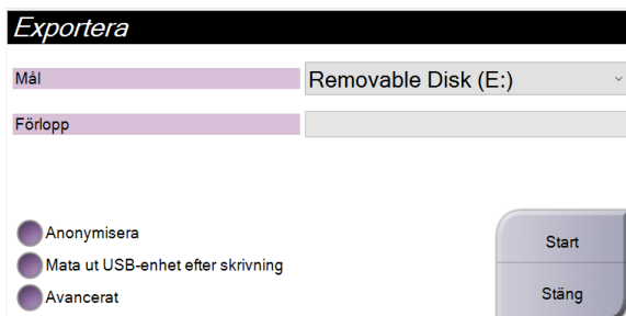
Figur 101: Skärmen Exportera
