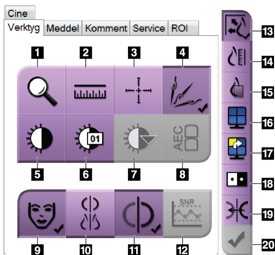
Figur 52: Bildgranskningsverktyg
