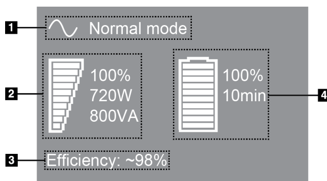
Figura 99: Pantalla LCD del UPS
