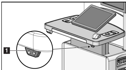
Figura 79: Panel de control de ajuste de altura
