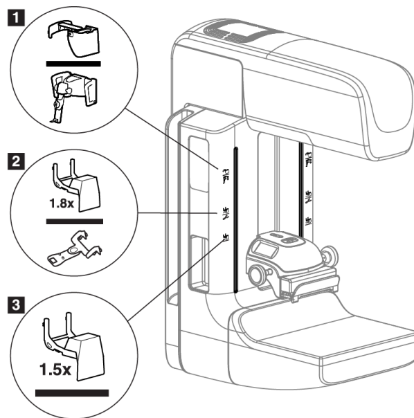
Abbildung 57: C-Bogenzubehör
