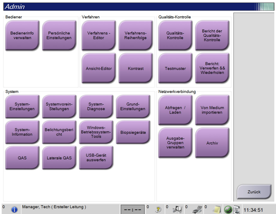
Abbildung 72: Bildschirm „Admin“
