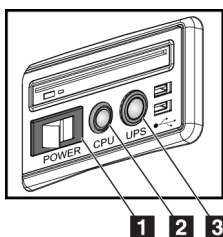
Abbildung 15: Netztasten an der Universal-Akquisitions-Workstation
