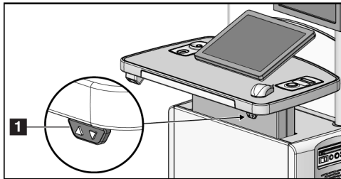
Abbildung 79: Bedienfeld Höhenregulierung
