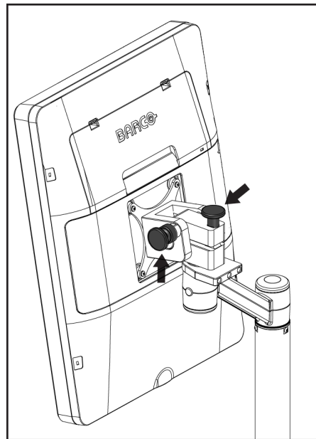
Abbildung 103: Knöpfe zur Verriegelung des drehbaren Monitors an der mobilen Universal-Akquisitions-Workstation (Serie II)
