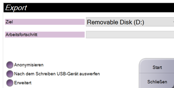
Abbildung 95: Bildschirm „Export“
