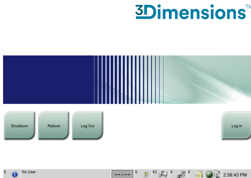
Abbildung 17: Startbildschirm
