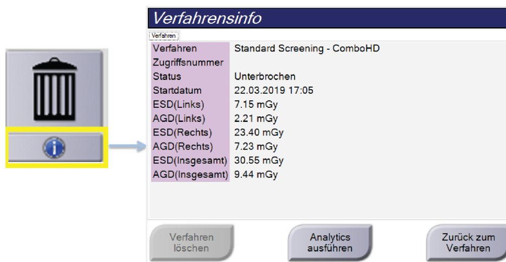
Abbildung 32: Dialogfeld „Verfahrensinfo“
