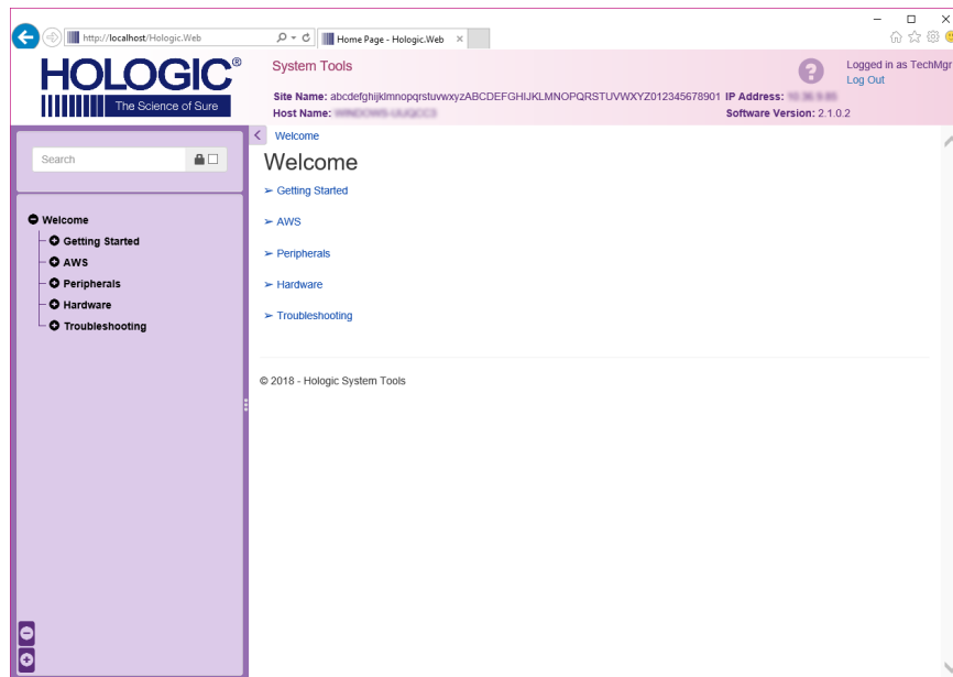
Abbildung 88: Bildschirm System-Einstellungen
