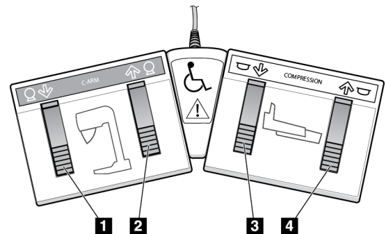
Abbildung 12: Zweifunktions-Fußschalter
