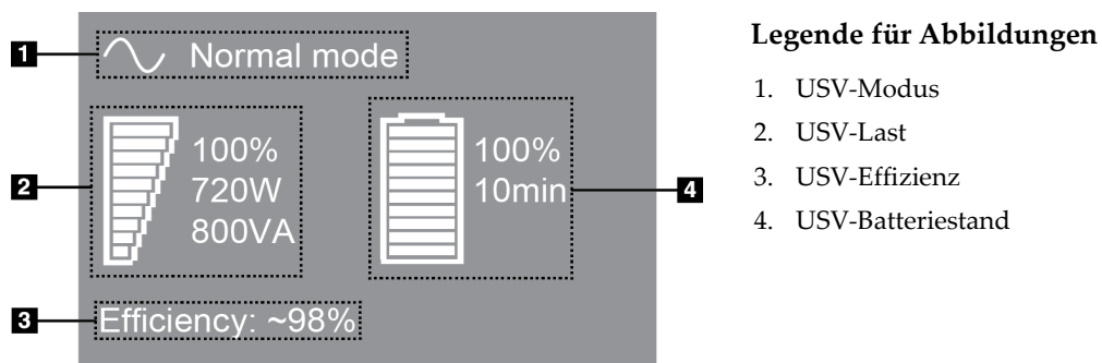
Abbildung 99: USV LCD-Display
