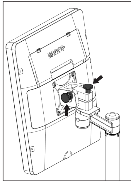
Εικόνα 110: Κουμπιά κλειδώματος περιστρεφόμενου μόνιτορ στον γενικό σταθμό εργασίας λήψης (σειρά II)
