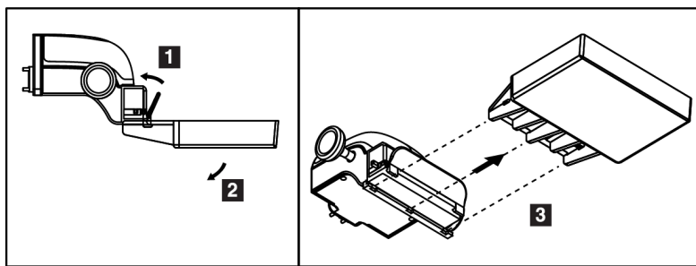
Εικόνα 67: Τρόπος αφαίρεσης πτερυγίου συμπίεσης
