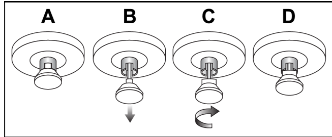
Εικόνα 108: Απελευθέρωση του κλειδώματος δίσκου από την κλειδωμένη (Α) στην ξεκλειδωτή θέση (D)
