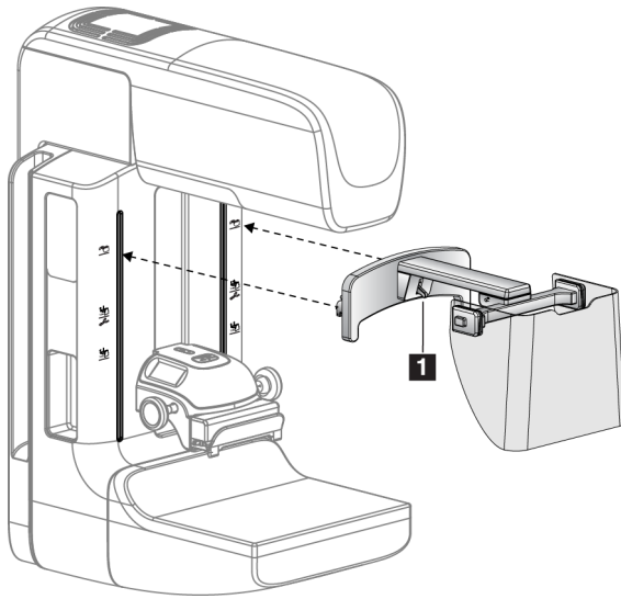
Kuva 63: Kasvosuojan asennus
