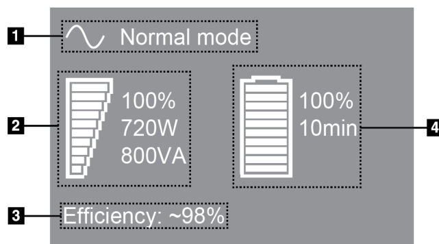
Kuva 106: UPS:n LCD-näyttö
