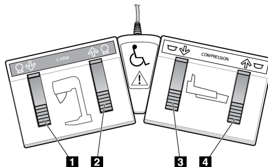
Kuva 11: Kaksoistoiminnon jalkakytkin
