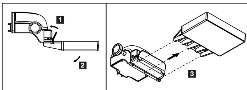
Kuva 67: Puristuslevyn poistaminen
