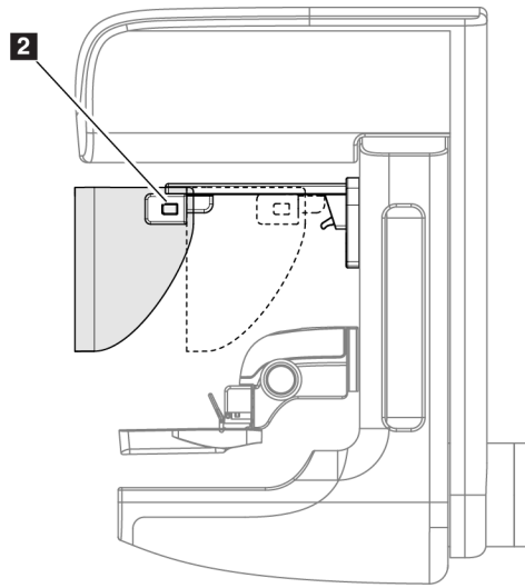
Kuva 64: Kasvosuojan käyttö
