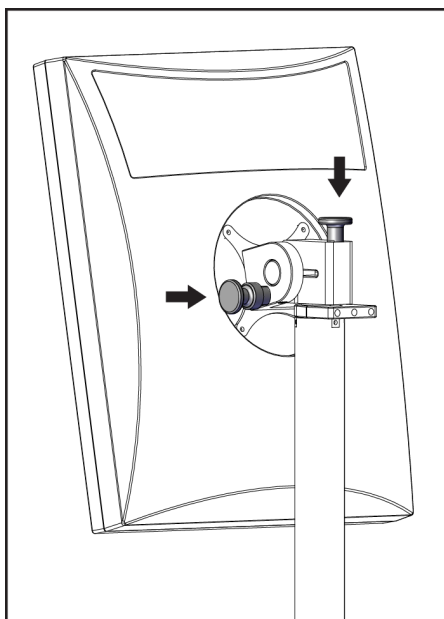
Figur 112: Låseknotter for den svingbare skjermen på den mobile universelle bildetakingsarbeidsstasjon (serie I)
