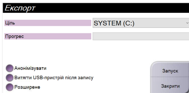
Рисунок 102: Екран «Експорт»
