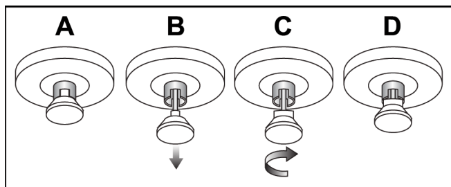
Рисунок 111: Переведення фіксатора полиці з заблокованого (A) у розблоковане (D) положення
