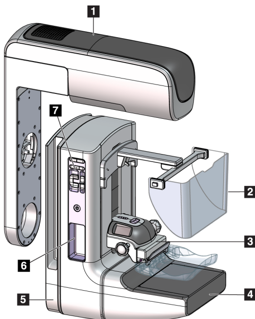
Рисунок 2: Огляд С-дуги
