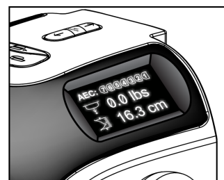
Рисунок 8: Дисплей компресійного пристрою
