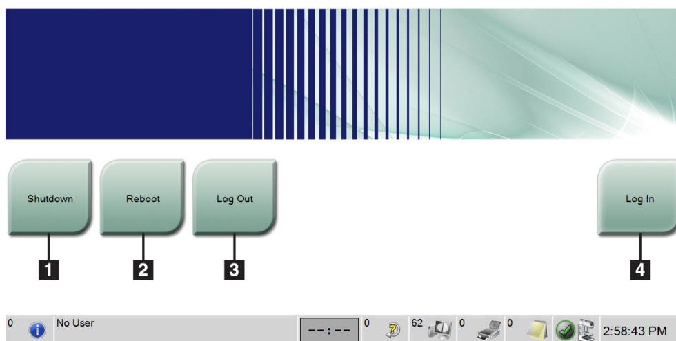
Рисунок 16: Екран запуску
