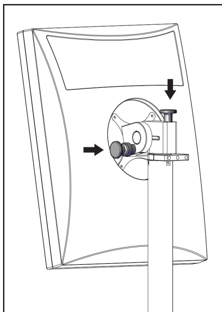
Figure 118 : Boutons de verrouillage de l'écran pivotant sur la station d'acquisition universelle mobile (série I)
