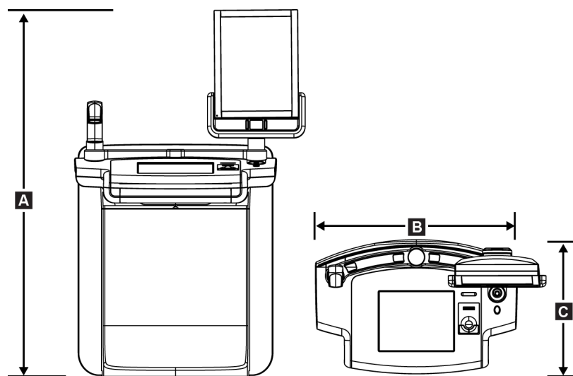
Figure 110 : Mesures de la station d'acquisition haut de gamme mobile
