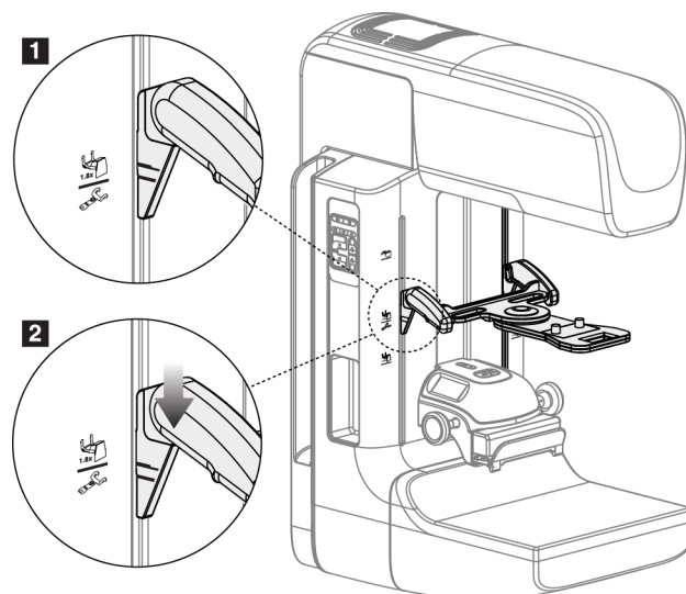
Figure 75 : Installation du dispositif réticulaire de localisation
