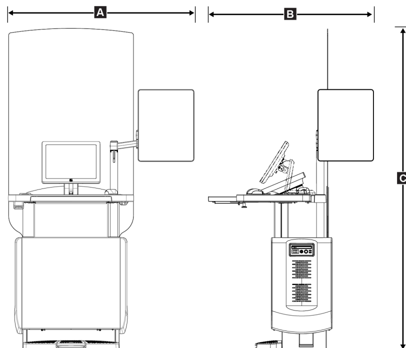
Figure 106 : Mesures de la station d'acquisition universelle
