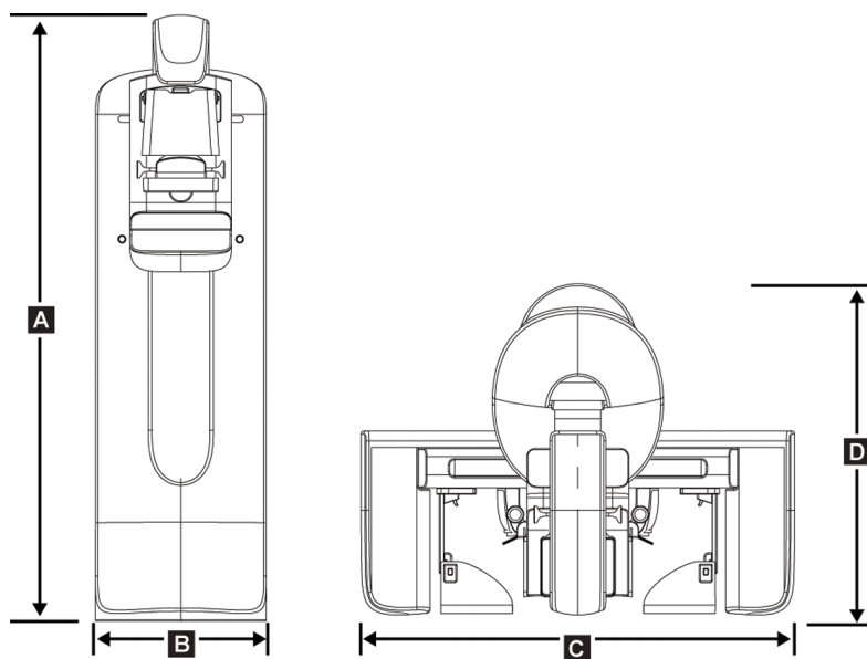
Figure 105 : Mesures du porte-tube (statif avec bras en C)
