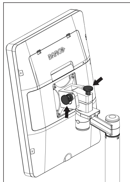
Figure 116 : Boutons de verrouillage de l'écran pivotant sur la station d'acquisition universelle mobile (série II)
