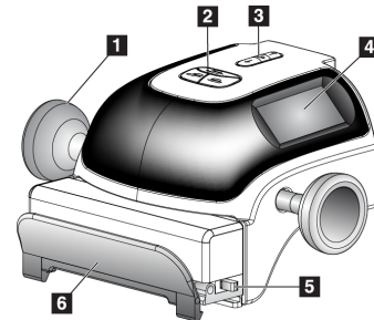
Figure 9 : Compresseur
