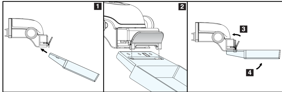
Figure 71 : Pour installer une pelote de compression
