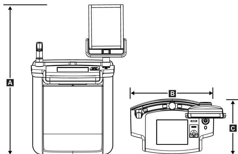
Figuur 114: Afmetingen Premium mobiel verwerfingswerkstation
