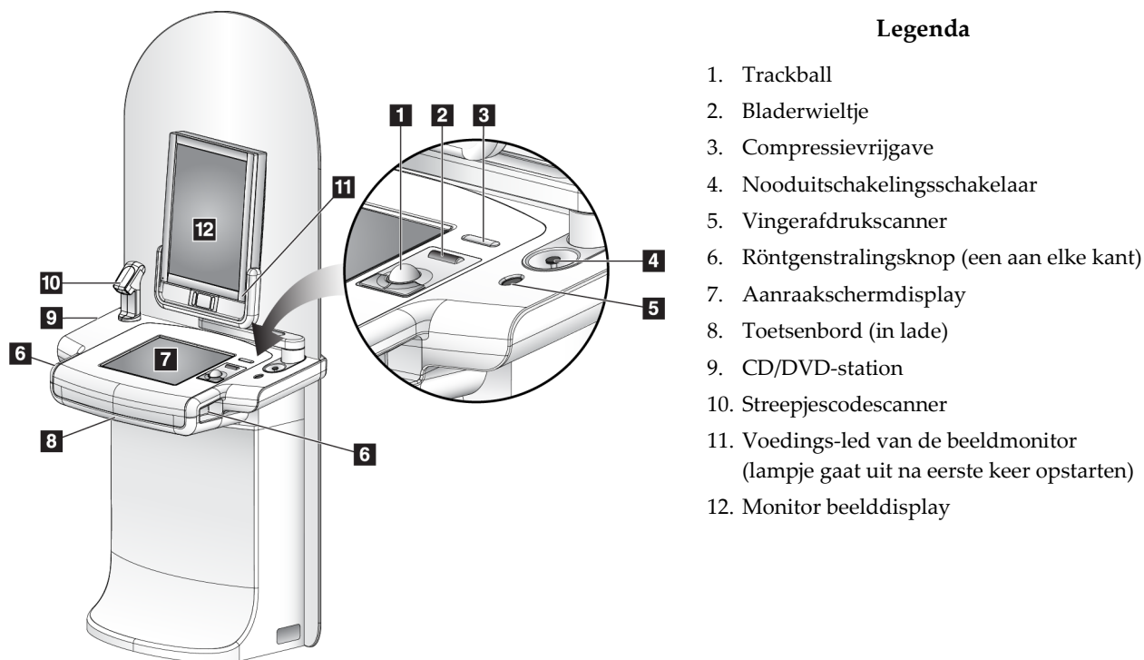
Figuur 13: Bedieningselementen en displays van het Premium verwervingswerkstation
