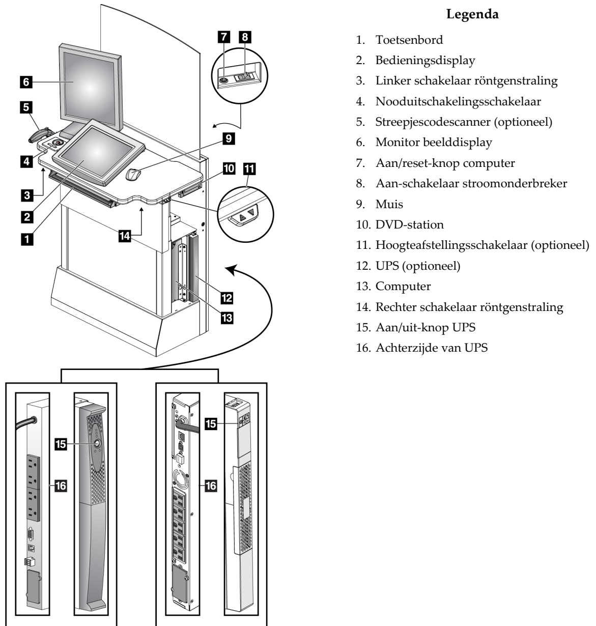
Figuur 14: Bedieningselementen en displays van het Standaard verwervingswerkstation
