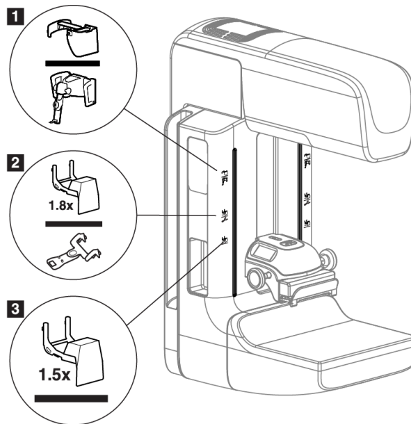
Figură 67: Accesoriiile brațului C
