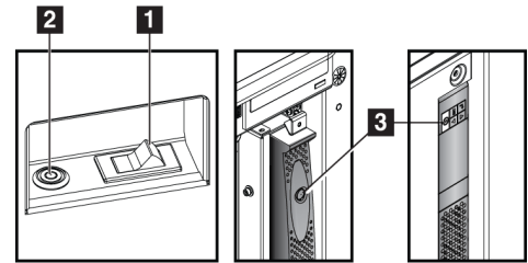
Figură 18: Butoanele de alimentare a stației de colectare standard
