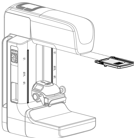
Figură 77: Instalarea și îndepărtarea dispozitivului cu vizor de amplificare
