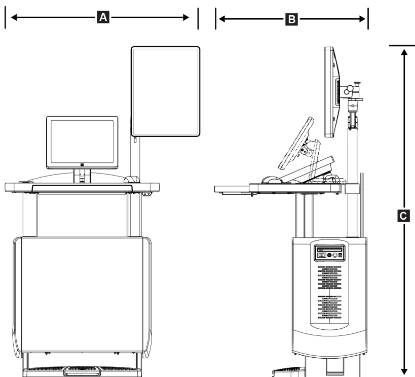
Figur 113: Mobil Universal bildetakingsarbeidsstasjon mål
