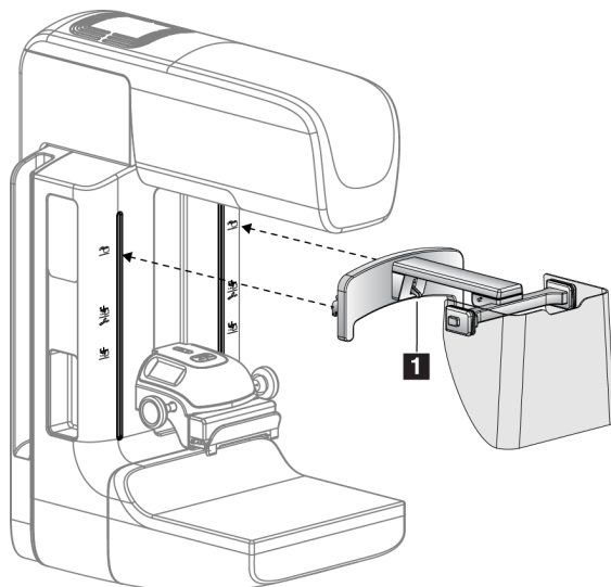
Figur 69: Ansiktsskjold installasjon
