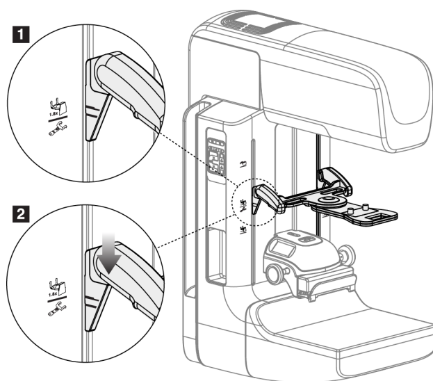
Figur 76: Installasjon av trådkorslokaliseringsenheten
