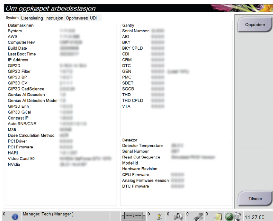
Figur 83: System-fanen på skjermbildet Om (bildetakingsarbeidsstasjon)
