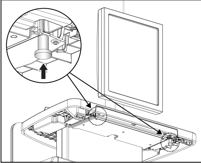
Şekil 116: Klavye Tepsisi Kilitleme Düğmesi (Sağ veya Sol Taraf) (Üniversal Görüntü Alım İş İstasyonu)
