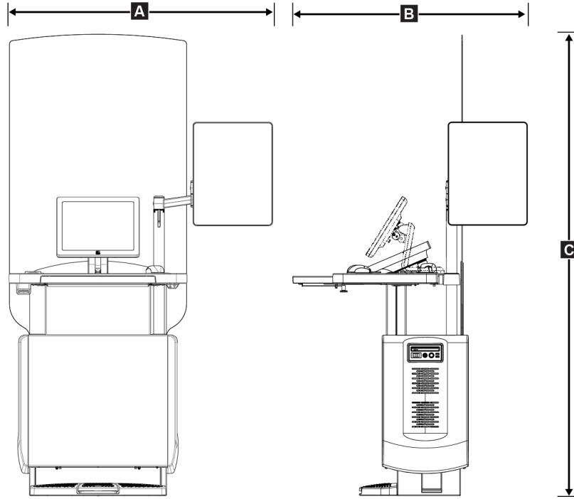
Şekil 110: Üniversal Görüntü Alım İş İstasyonu Ölçüleri
