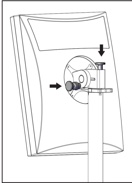
Şekil 122: Mobil Üniversal Görüntü Alım İş İstasyonundaki Döner Monitör Kilit Düğmeleri (seri I)
