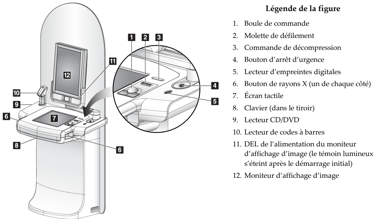
Figure 14 : Commandes et affichages de la station d'acquisition haut de gamme
