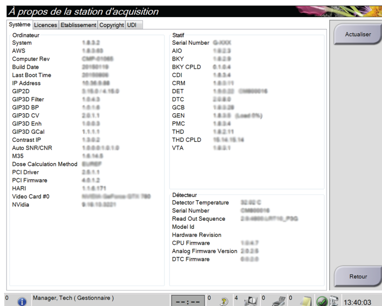
Figure 79 : Onglet Système de l'écran À propos de (station d'acquisition)
