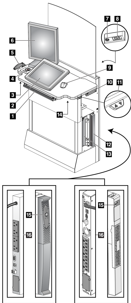
図15: 標準画像取り込みワークステーションの制御とディスプレイ
