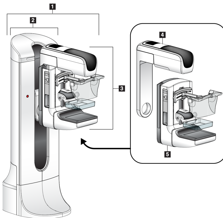
図 1: Selenia® Dimensions® システムのチューブスタンド
