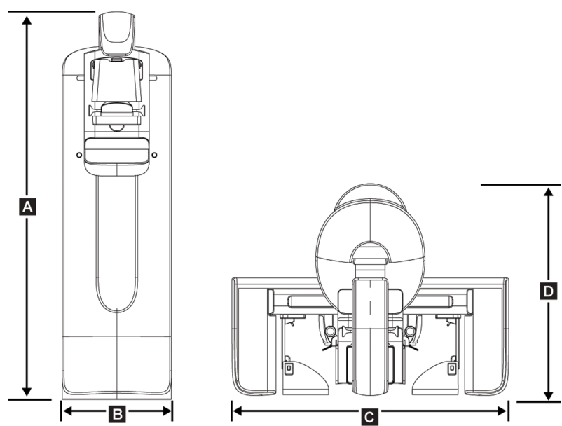
図102: チューブスタンド (C アーム付きガントリー) 寸法
