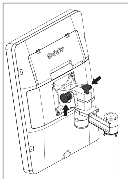
図116: 車載用汎用型画像取り込みワークステーション（シリーズII）の上に配置された画像表示モニター用の回転式ロックノブ
