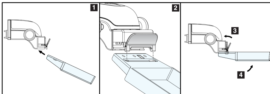
Figura 68: Como instalar uma pá de compressão
