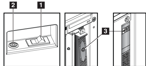
Figuur 19: Aan/uit-knoppen Standaard verwervingswerkstation
