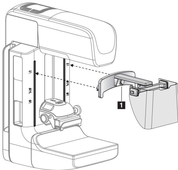
Figuur 68: Installatie van het gezichtsschermbewakingspaneel
