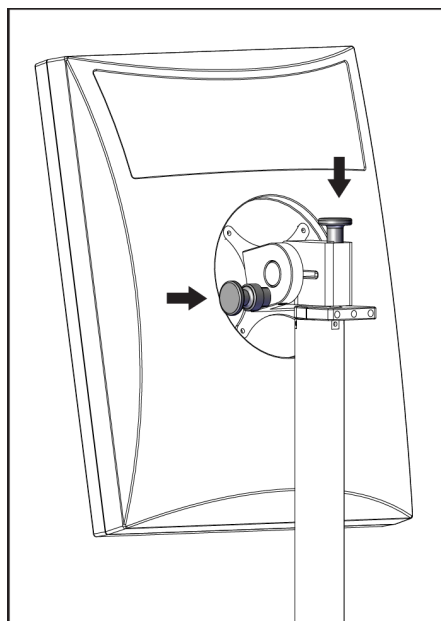
Figuur 118: Vergrendelingsknoppen zwenkbare monitor op het mobiele Universele verwervingswerkstation (serie I)
