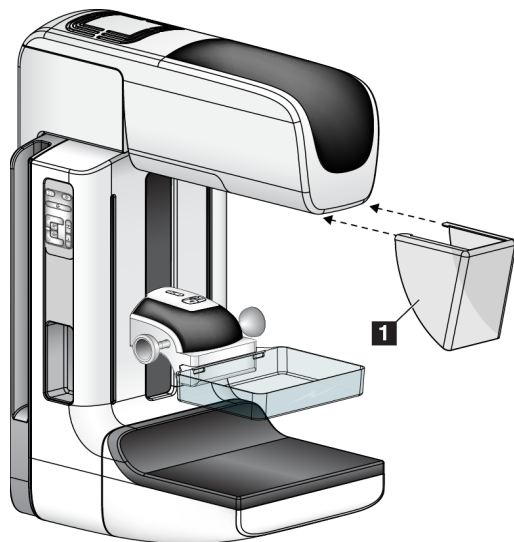
Figuur 70: Het conventionele gezichtsscherf installeren
