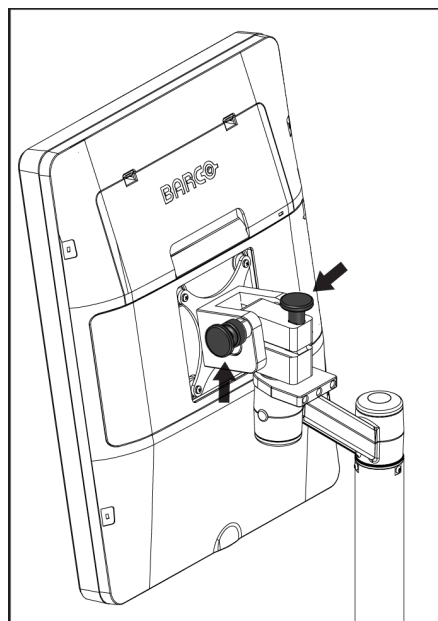
Figuur 119: Vergrendelingsknoppen zwenkbare monitor op het mobiele Universele verwervingswerkstation (serie II)
