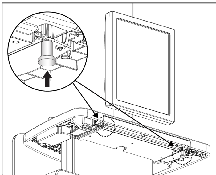
Figuur 112: Vergrendelingsknop toetsenbordlade, rechts of links (Universeel verwerfingswerkstation)
