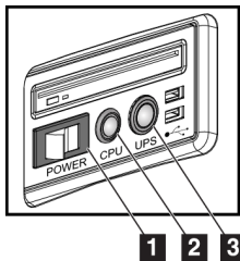
Figuur 17: Aan/uit-knoppen Universeel verwervingswerkstation
