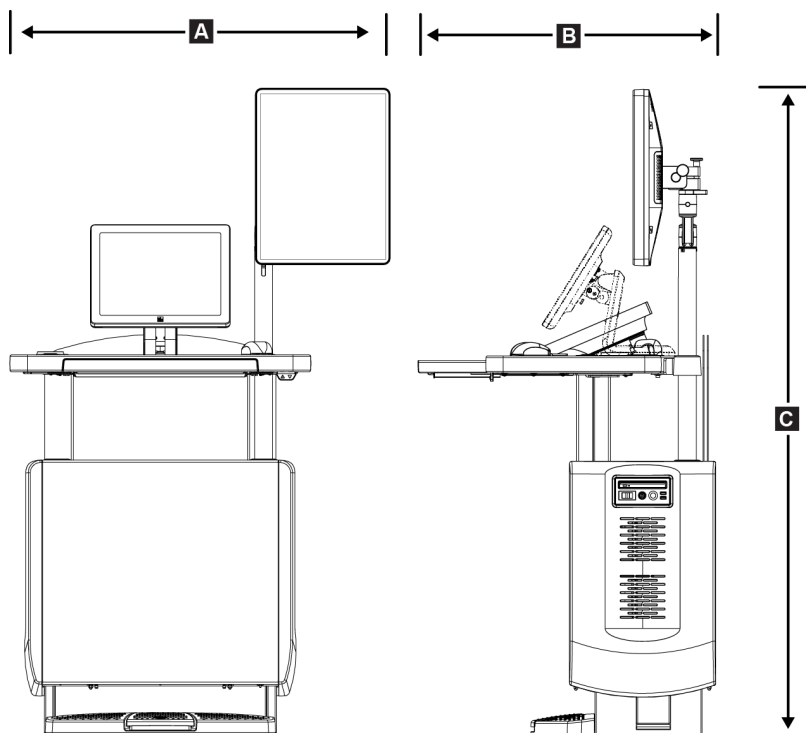
Figuur 109: Afmetingen mobiel universeel verwervingswerkstation
