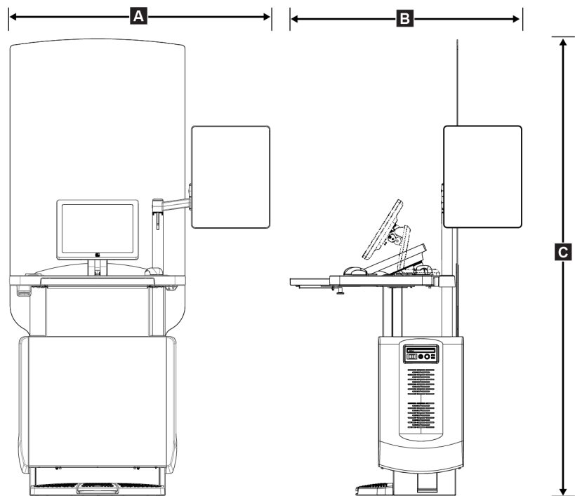
Figuur 106: Afmetingen universeel verwervingswerkstation
