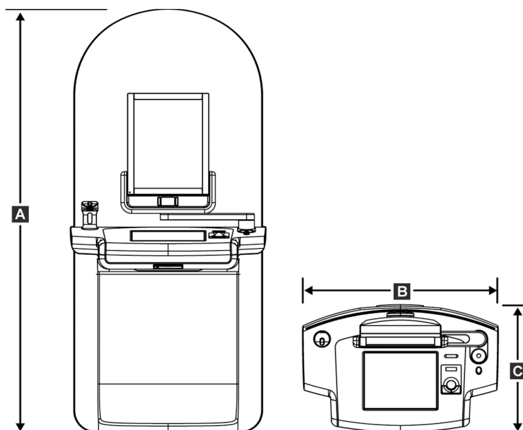
Figuur 107: Afmetingen Premium verwervingswerkstation
