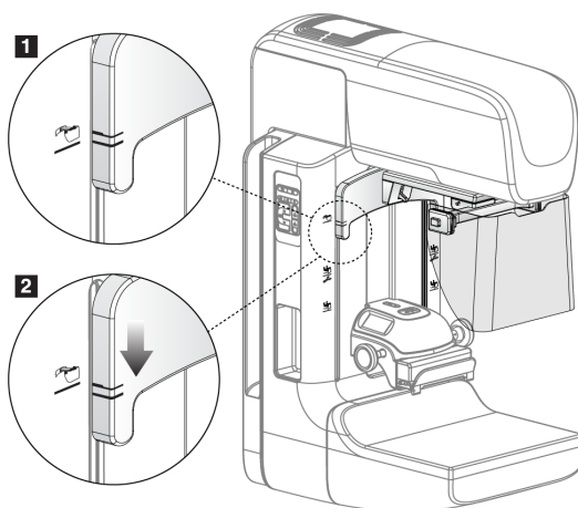
Figuur 67: Het intrekbare gezichtsschermbuitlijnen met de C-arm
