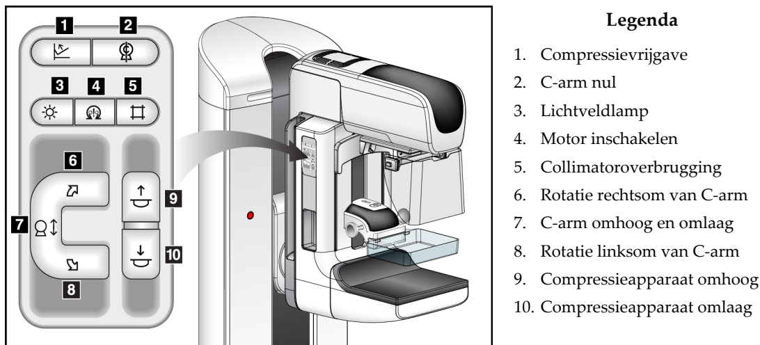
Figuur 23: Bedieningspaneel op C-arm (linkerkant afgebeeld)
