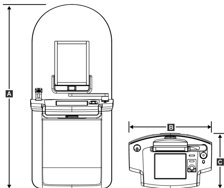
Kuva 107: Erikoismallisen kuvaustyöaseman mitat
