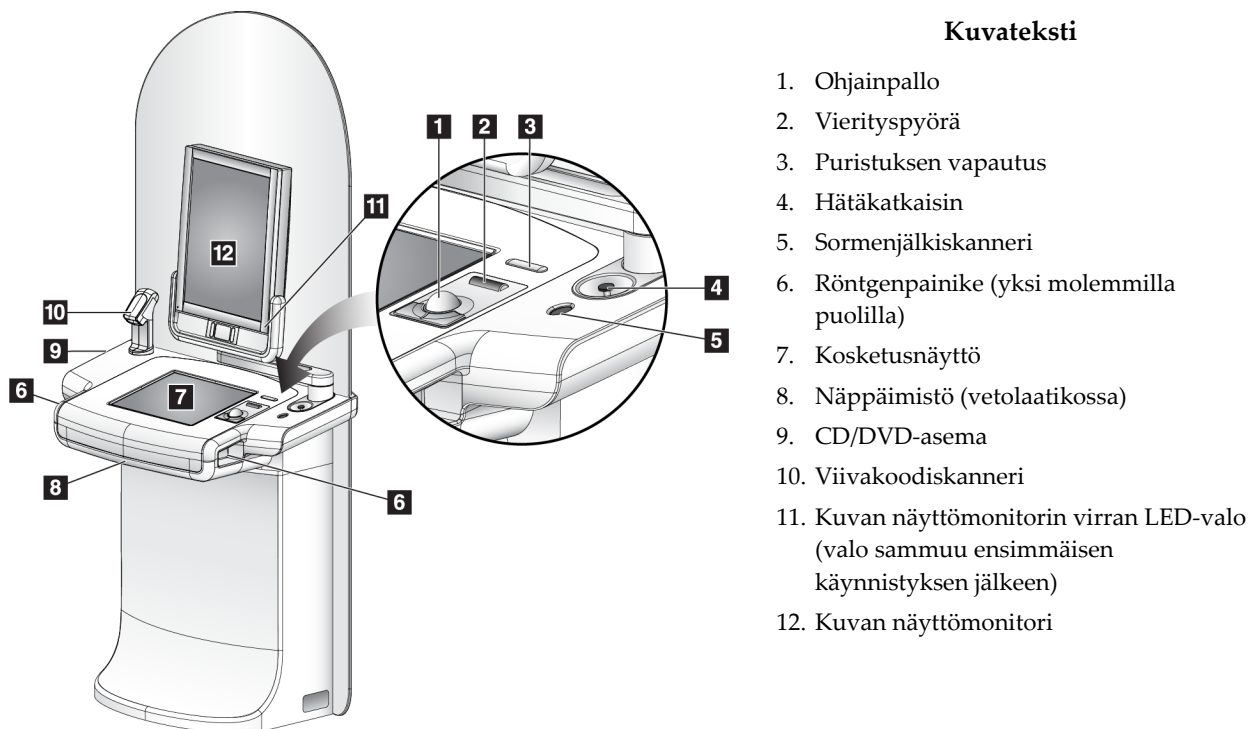
Kuva 14: Erikoismallisen kuvaustyöaseman ohjaimet ja näytöt
