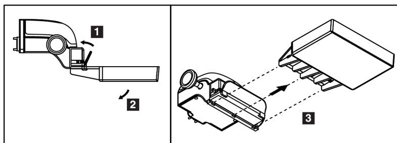
Kuva 72: Puristuslevyn poistaminen
