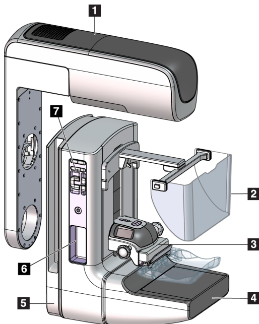
Kuva 2: C-kaarilaitteen yleiskuvaus
