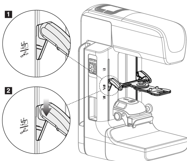
Kuva 75: Paikantavan hiusristilaitteen asentaminen
