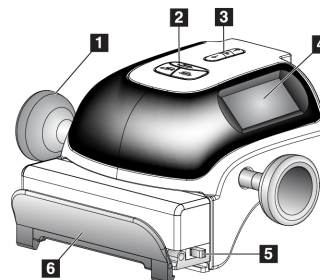
Kuva 9: Puristuslaite
