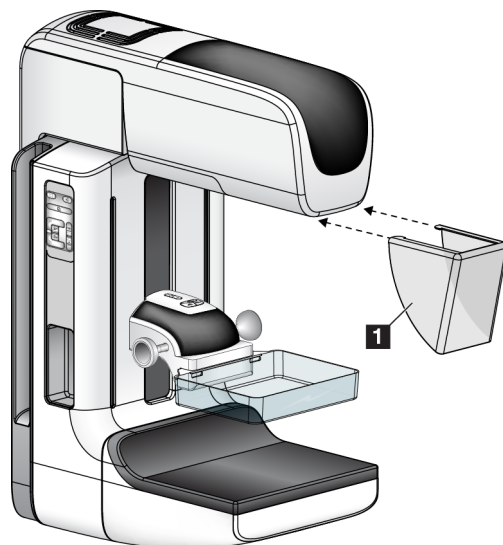
Kuva 70: Perinteisen kasvosuojan asentaminen
