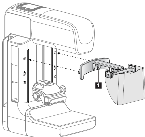
Kuva 68: Kasvosuojan asennus
