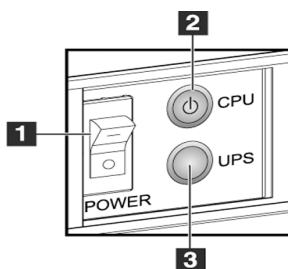
Kuva 26: Erikoismallisen kuvaustyöaseman virtapainikkeet
