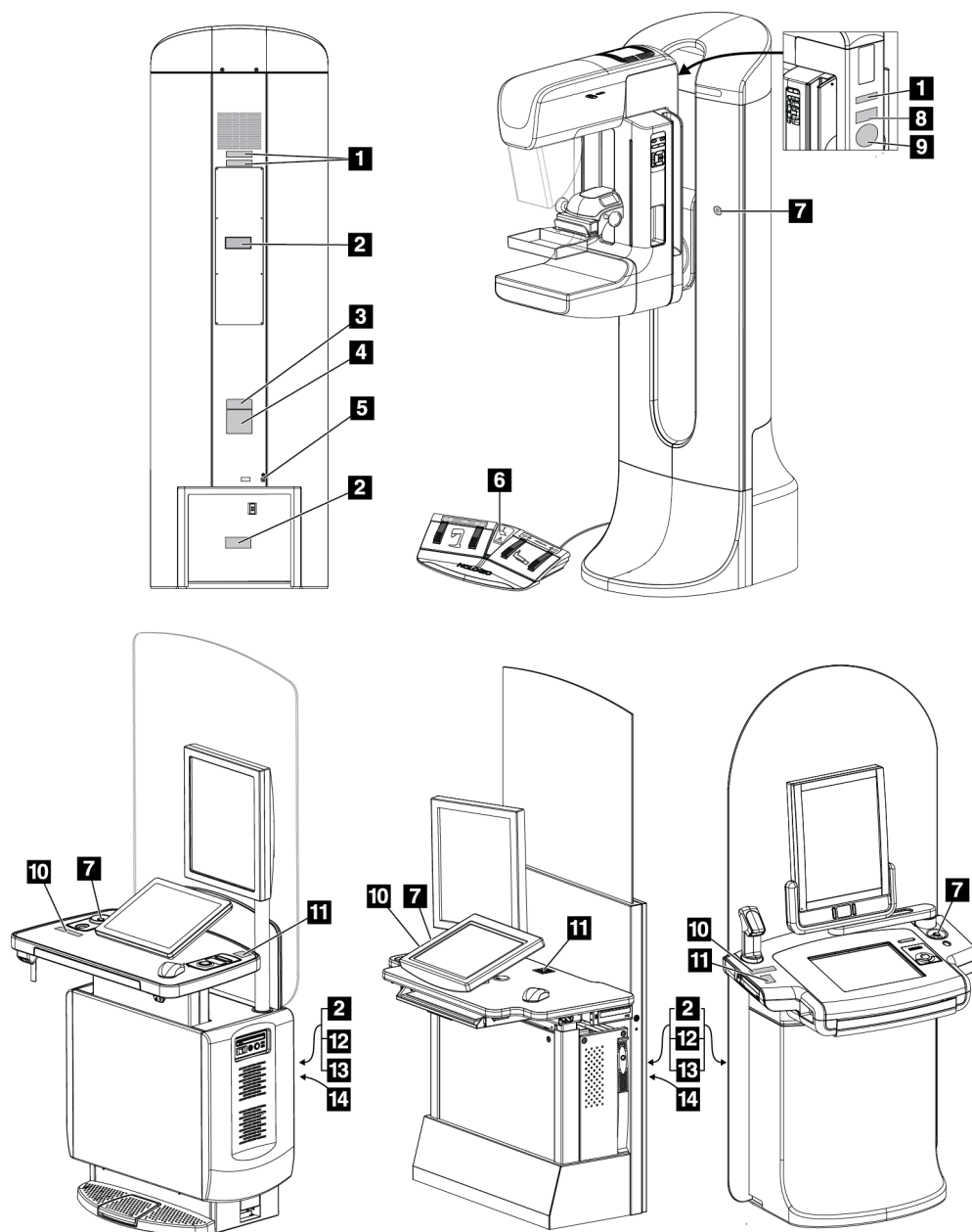
Figur 5: Etikettplasseringer
