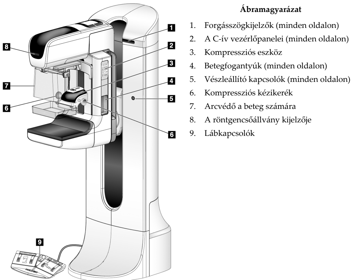
Ábra 7: Röntgensóállvány-vezérlők és -jelzők
