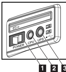
Ábra 25: Az univerzális felvételi munkaállomás tápkapcsoló gombjai
