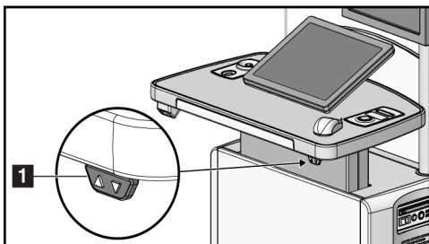
Ábra 94: Magasságbeállítás vezérlőpanele
