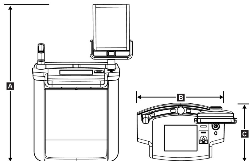
Ábra 110: Prémium, mobil felvételkedészítő munkaállomás méretei
