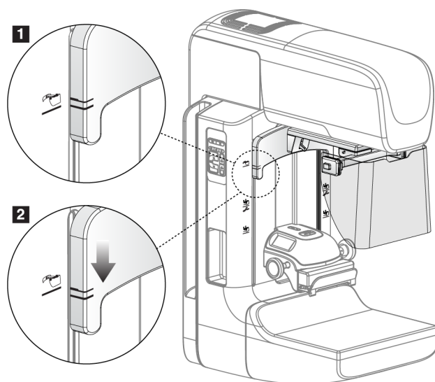
Ábra 67: A visszahúzható arcvédő pajzs C-ívhez igazítása
