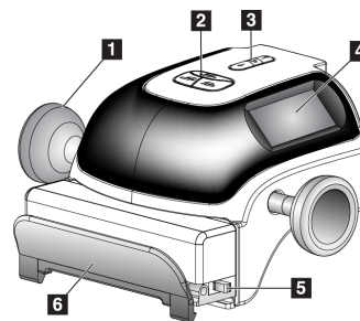
Ábra 9: Kompressziós eszköz
