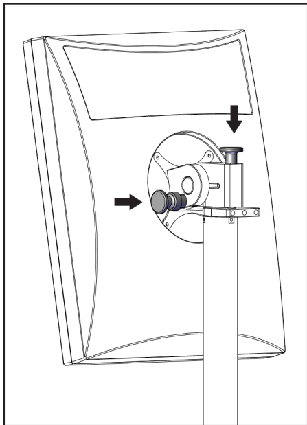
Ábra 115: Forgómonitor zárógombok a mobil univerzális felvételkedszítő munkaállomáson (I. sorozat)
