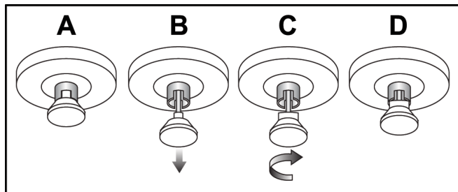
Ábra 117: Tálcazár kioldása zárolt (A) helyzetből nyitott (D) helyzetbe
