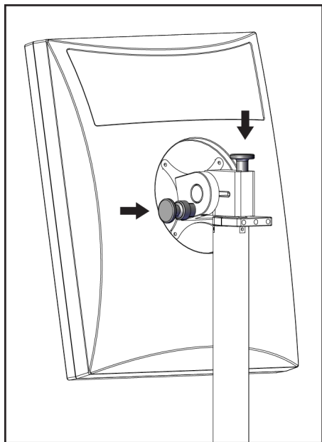
Obrázok 115: Blokovacie kolíky otočného monitora na mobilnej univerzálnej snímacej pracovnej stanici (séria I)
