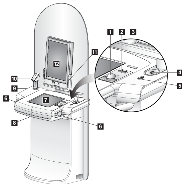
Obrázok 14: Ovládacie prvky a displeje prémiovej snímačej pracovnej stanice
