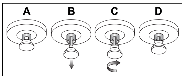
Obrázok 114: Uvoľnenie blokovania zásuvky zo zamknutej polohy (A) do odomknutej polohy (D)
