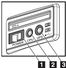
Rycina 17: Przyciski zasilania uniwersalnej stacji roboczej akwizycji
