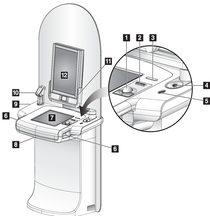
Rycina 14: Elementy sterujące i wyświetlacze zaawansowanej stacji roboczej akwizycji
