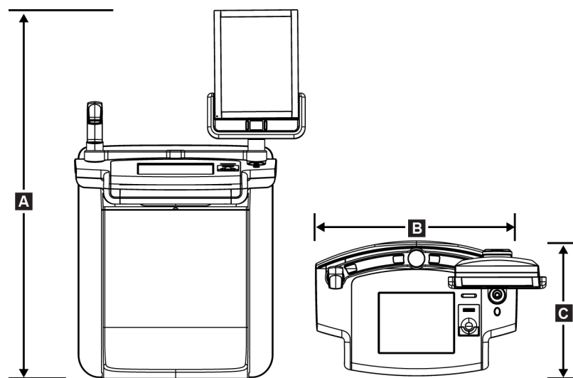
Rycina 110: Wymiary mobilnej zaawansowanej stacji roboczej akwizycji
