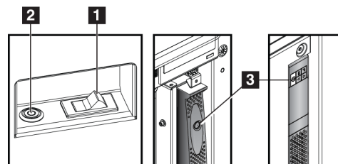
Figura 26: Botões de alimentação na Estação de Trabalho de Aquisição Padrão
