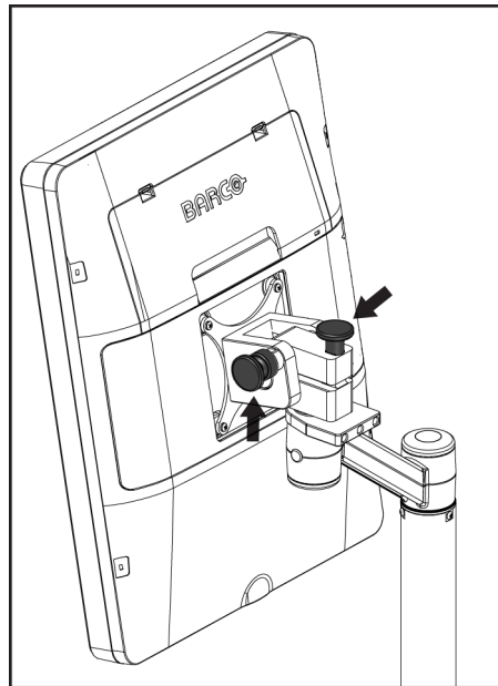
Figura 120: Botões de bloqueio do monitor articulado na Estação de Trabalho de Aquisição Universal Móvel (série II)
