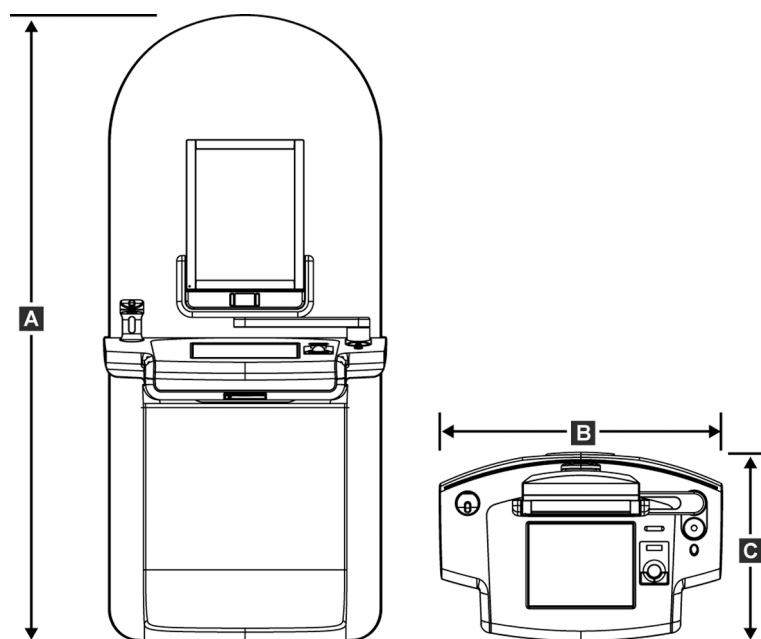
Figura 111: Medidas da Estação de Trabalho de Aquisição Superior
