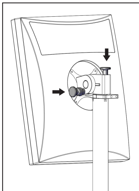
Figura 122: Botões de bloqueio do monitor articulado na Estação de Trabalho de Aquisição Universal móvel (série I)
