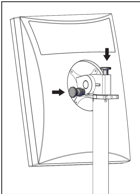
Figura 119: Botões de bloqueio do monitor articulado na Estação de Trabalho de Aquisição Universal Móvel (série I)
