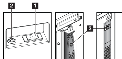
Figura 18: Botões de alimentação na Estação de Trabalho de Aquisição Padrão
