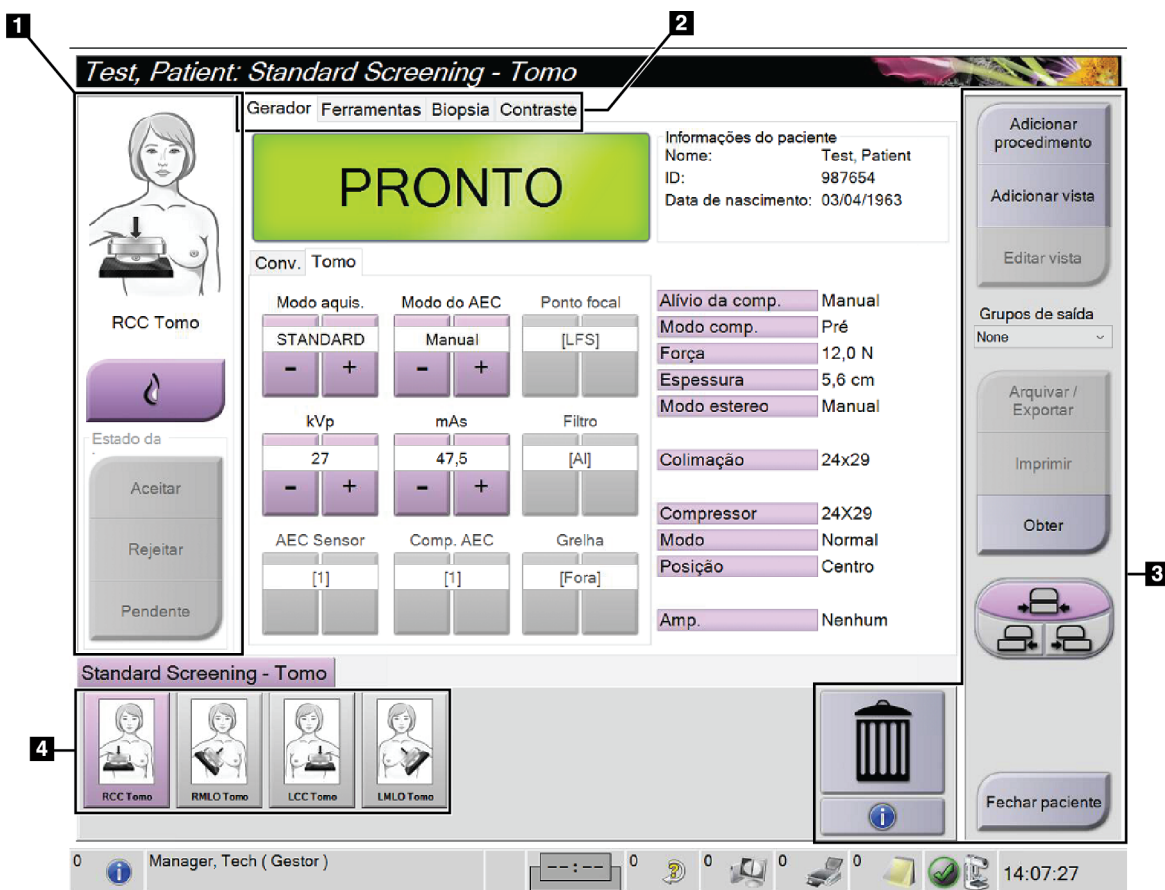
Figura 35: Ecrã do procedimento
