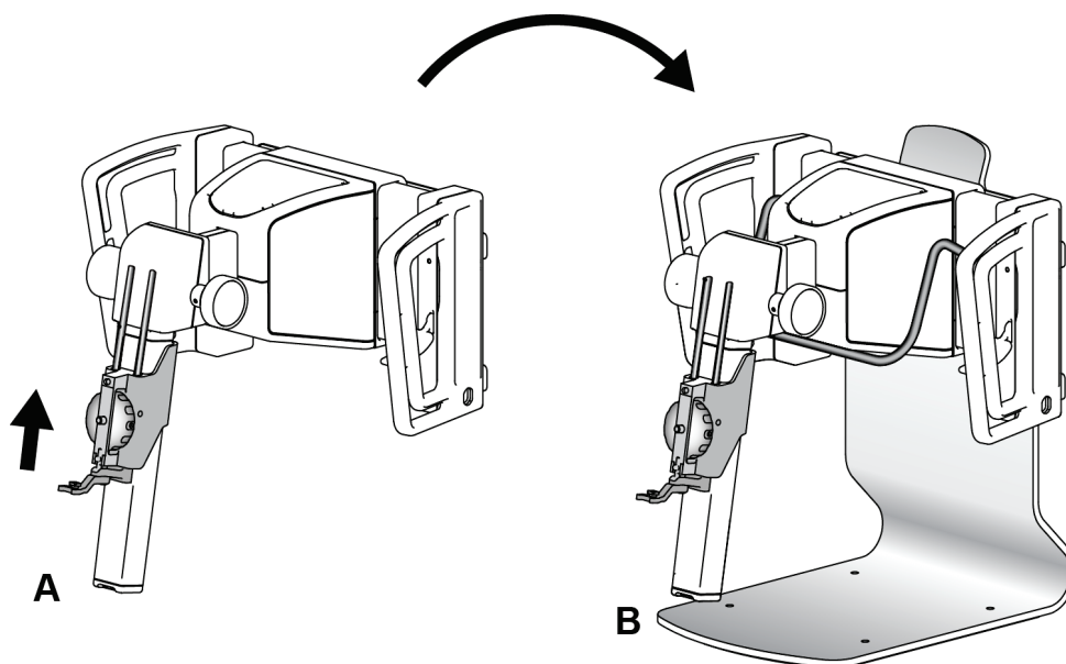
Figur 33: Affirm-systemets bordsstativ
