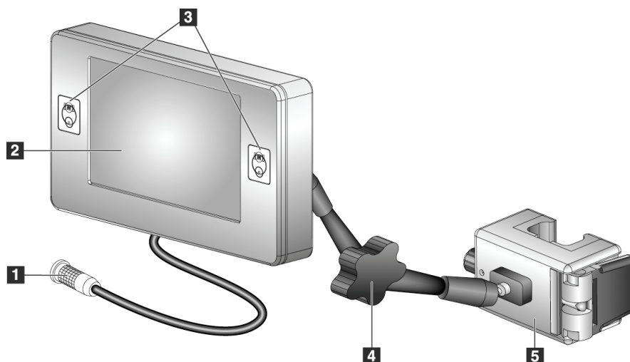
Figur 7: Biopsikontrollmodul
