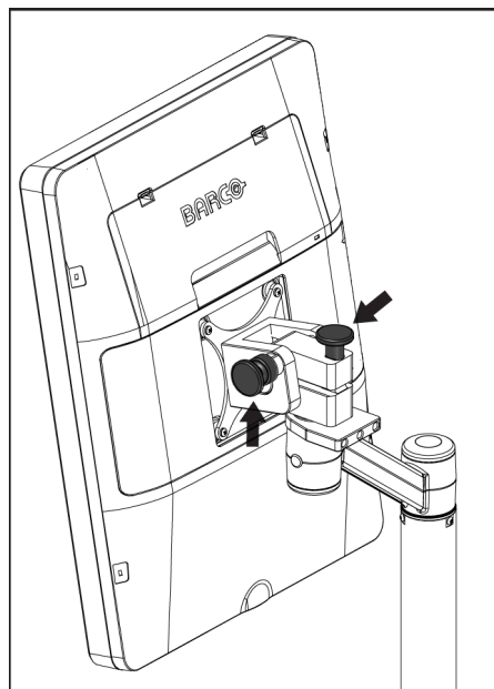
Abbildung 109: Knöpfe zur Verriegelung des drehbaren Monitors an der mobilen Universal-Akquisitions-Workstation (Serie II)
