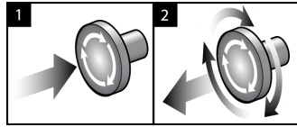
Abbildung 20: Die Not-Aus-Funktion
