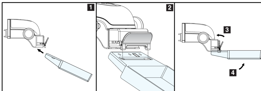
Abbildung 65: So installieren Sie eine Kompressionsplatte
