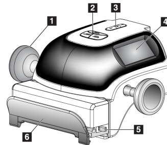
Abbildung 8: Kompressionsvorrichtung
