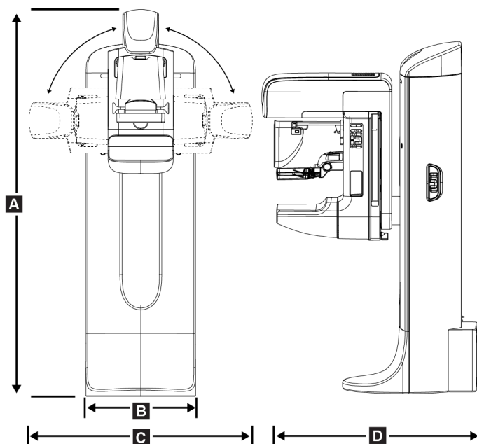
Abbildung 99: Abmessungen Säulenstativ (Gantry mit C-Bogen)
