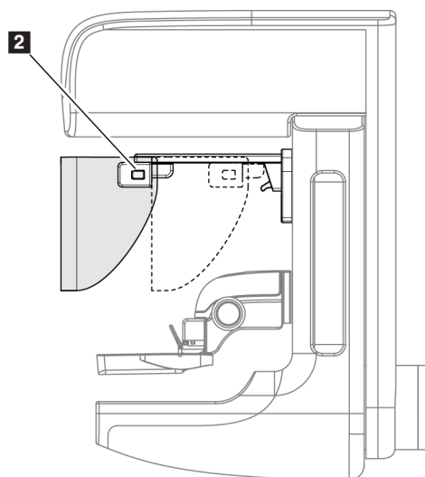
Abbildung 63: Bedienung des Gesichtsschutzes
