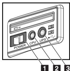
Figura 21: Botones de encendido de la estación de trabajo de adquisición universal
