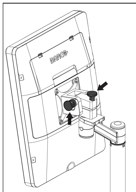
Figura 106: Perillas de bloqueo del monitor basculante en la estación de trabajo de adquisición universal móvil (serie II)
