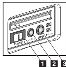
Figura 15: Botones de alimentación de la estación de trabajo de adquisición universal
