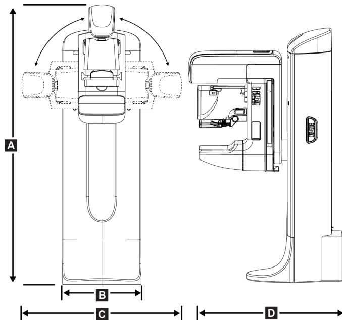
Kuva 99: Putkiteline (gantry ja C-kaari) Mitat
