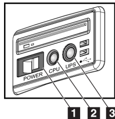
Kuva 21: Universaalin kuvauksen työaseman virtapainikkeet
