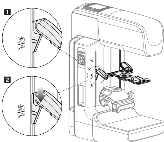
Kuva 69: Paikantavan hiusristilaitteen asentaminen
