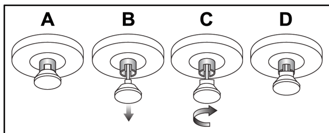
Kuva 107: Alustan lukon vapautus lukitusta (A) lukitsemattomaan (D)
