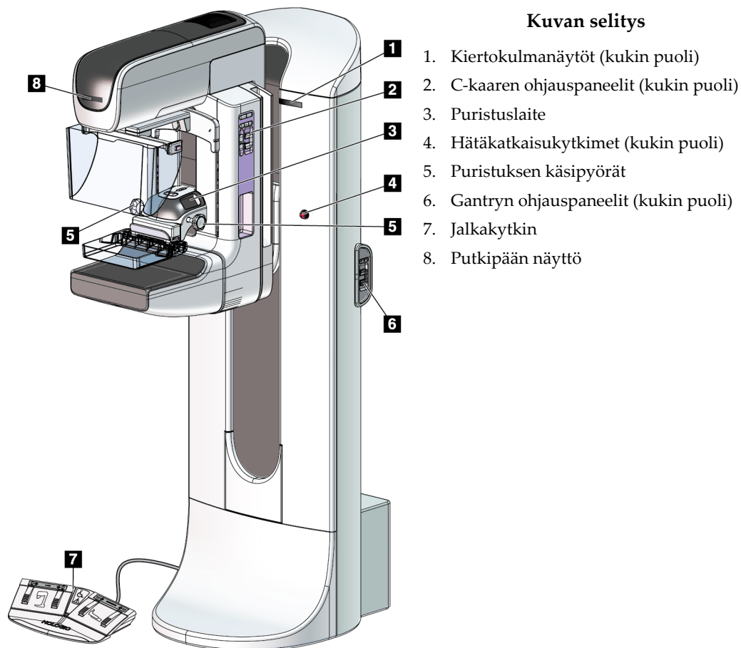
Kuva 6: Putkitelineen ohjauslaitteet ja ilmaisimet
