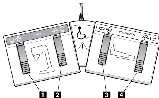
Kuva 12: Kaksoistoiminnon jalkakytkin
