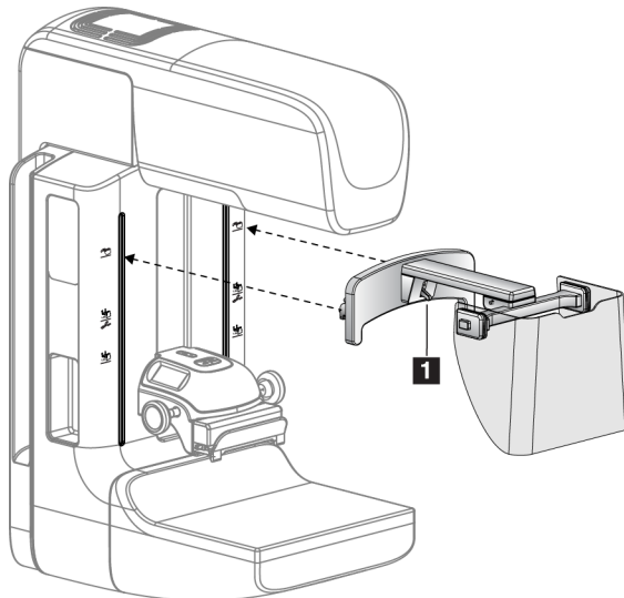
Kuva 62: Kasvosuojan asennus
