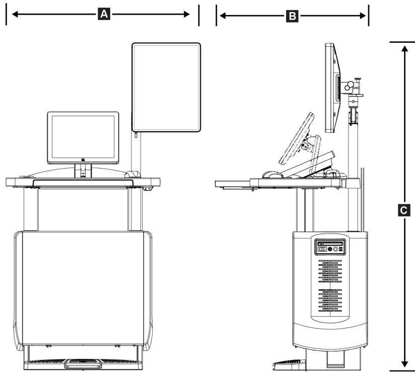
Kuva 101: Liikutettavan universaalin kuvauksen työaseman mitat
