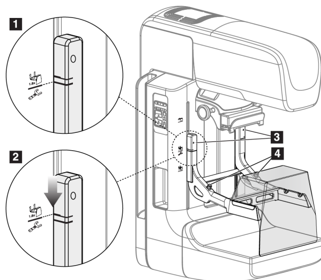
Kuva 68: Suurennustelineen asentaminen
