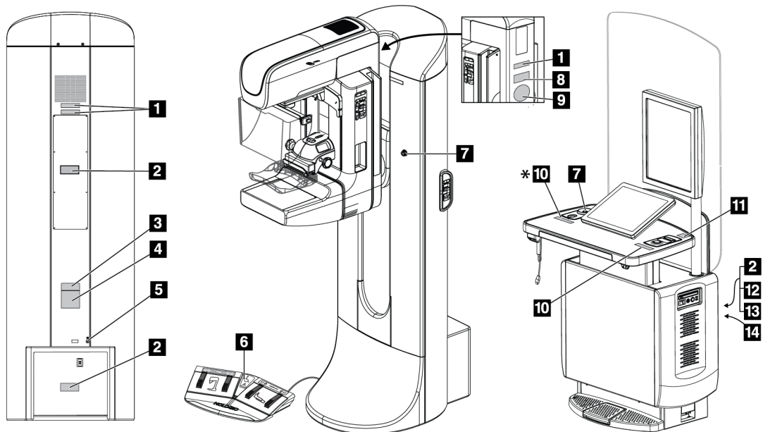
Kuva 4: Etiketin sijainnit
