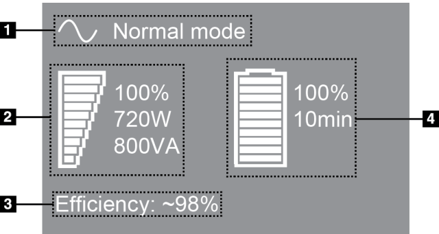
Figura 102: Pantalla LCD del UPS
