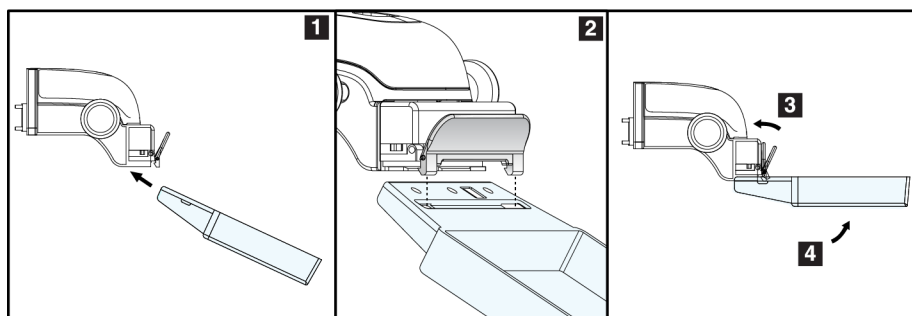
Figura 65: Instalación de la pala de compresión
