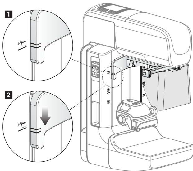
Figură 61: Alinierea scutului pentru față retractabil pe brațul C
