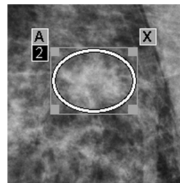
Figura 64: Ellipse (Elipsă)
