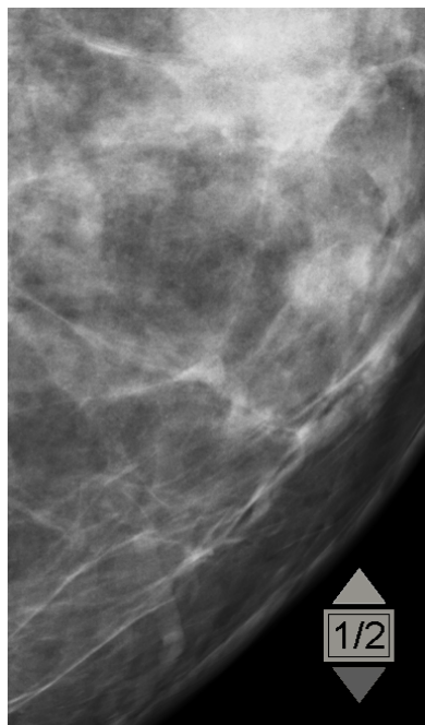
Figura 52: Imagine originală
