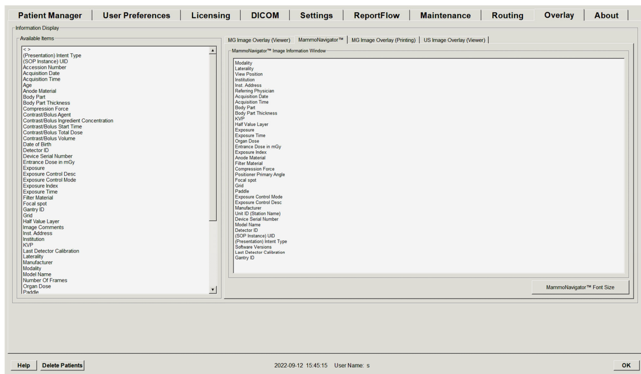
Figura 120: Fila MammoNavigator
