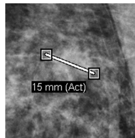
Figura 66: Measurement (Măsurătoare)
