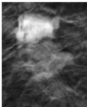
Figura 59: PeerView dezactivat
