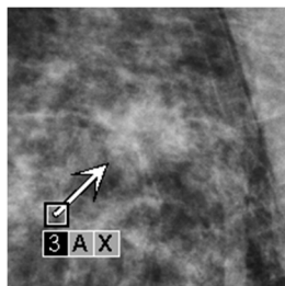
Figura 65: Arrow (Săgeată)
