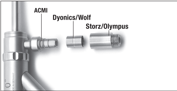
KUVA 4. VALOPYLVÄSSOVITTIMET
