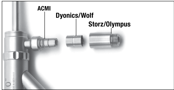
图 4.灯柱适配器
