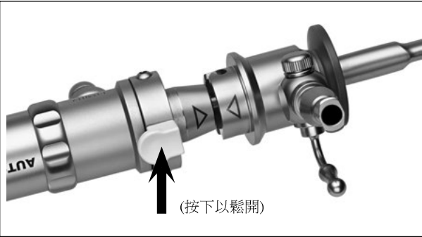
圖 2. 固定護套
