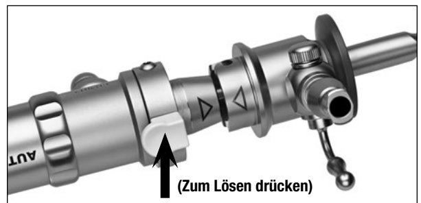
ABBILDUNG 2. SICHERE HÜLLE
