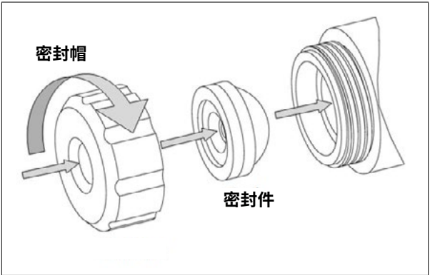
图 3.密封件安装
