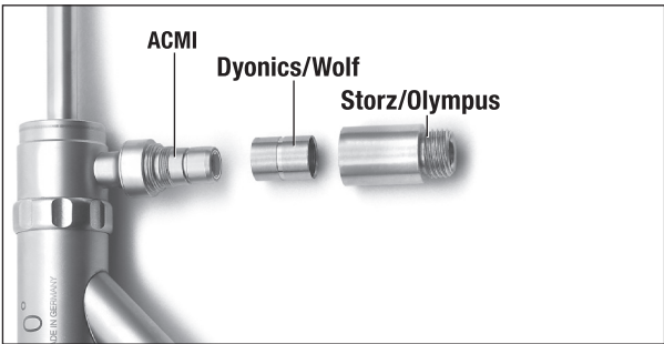
AFBEELDING 4. LICHTPOOTADAPTERS
