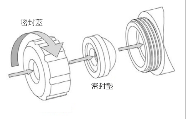
圖 3. 安裝密封墊
