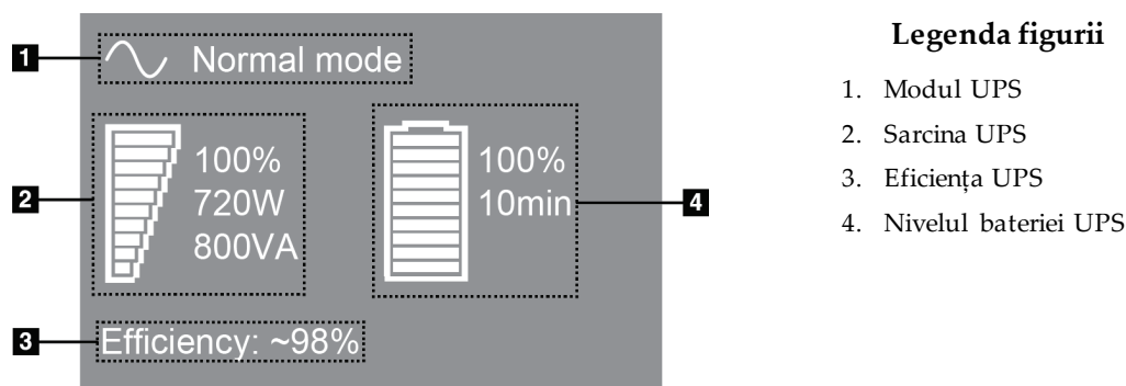
Figură 102: Ecranul LCD UPS
